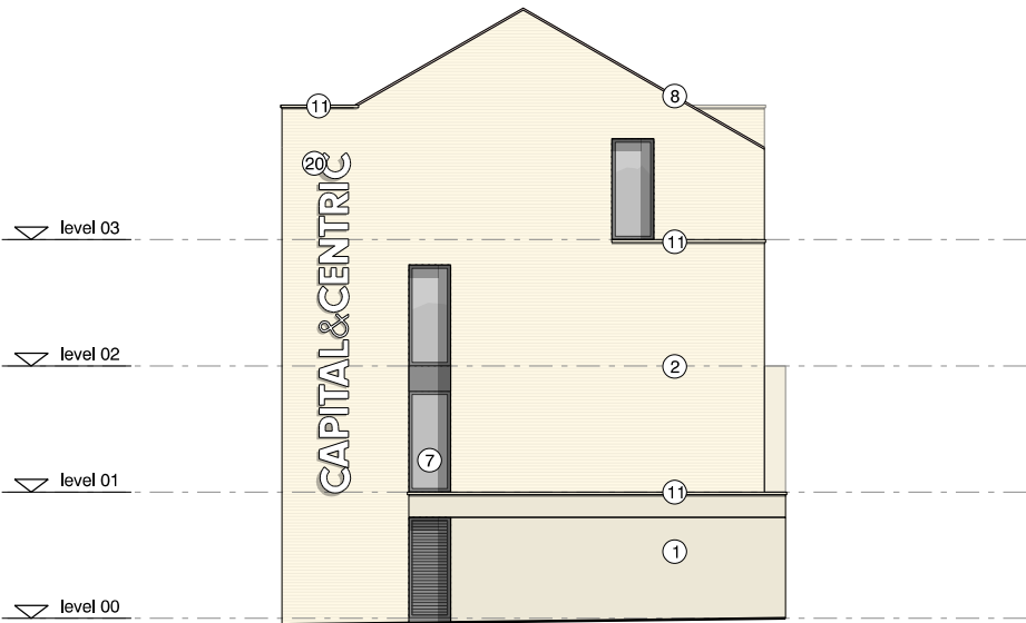
elevation 04
