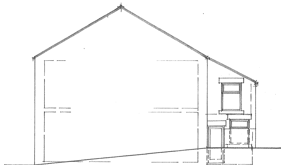
SIDE ELEVATION / N.E.
