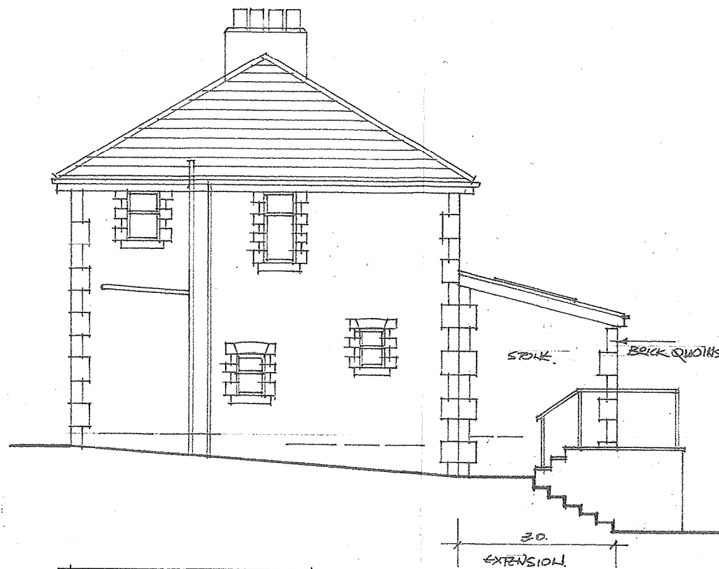
SIDE ELEVATION N.E.
