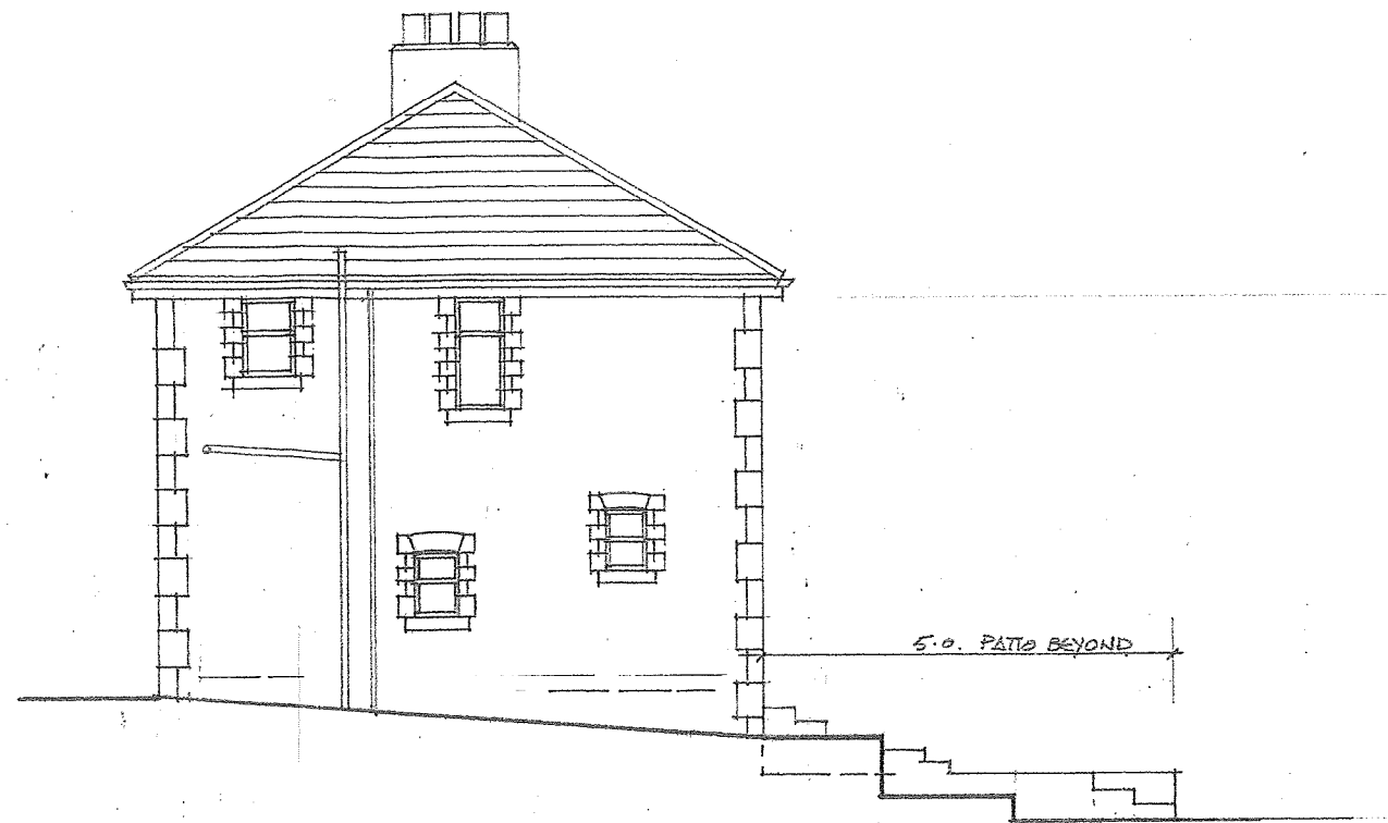
SIDE ELEVATION N.E.
