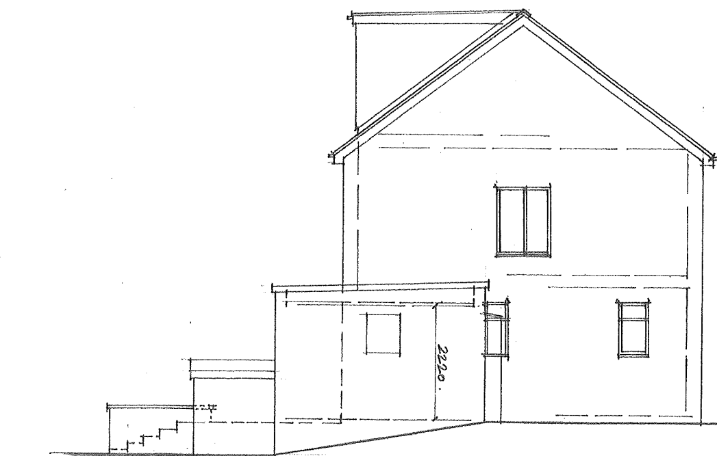
SIDE ELEVATION H.W.
