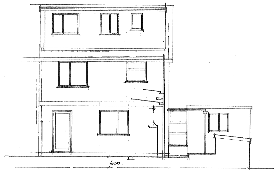
REAR ELEVATION N.E.
