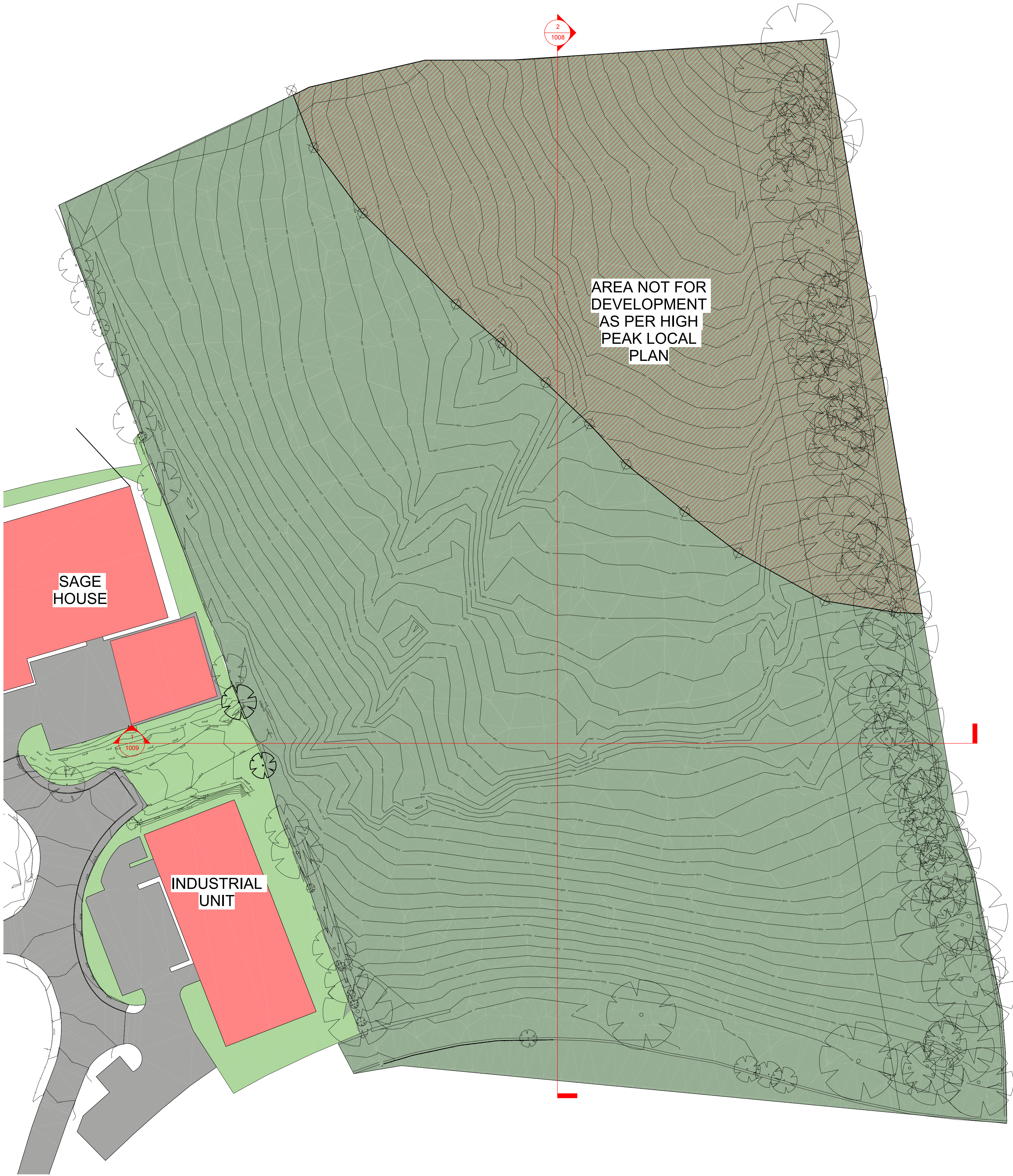
Site Block Plan Existing 1 : 500
