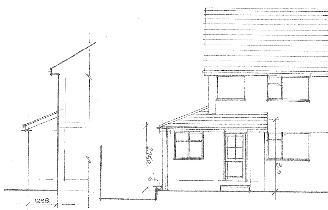
SIDE ELEVATION / N.W.
