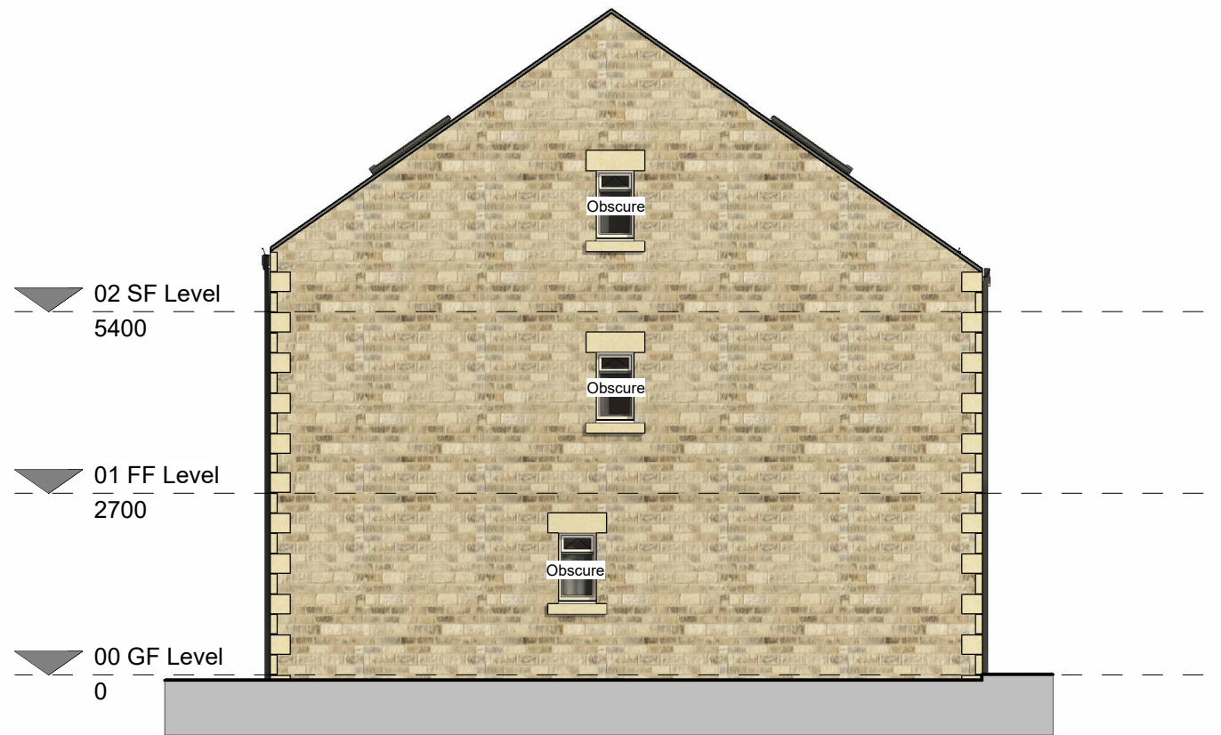
Left 1 : 100
