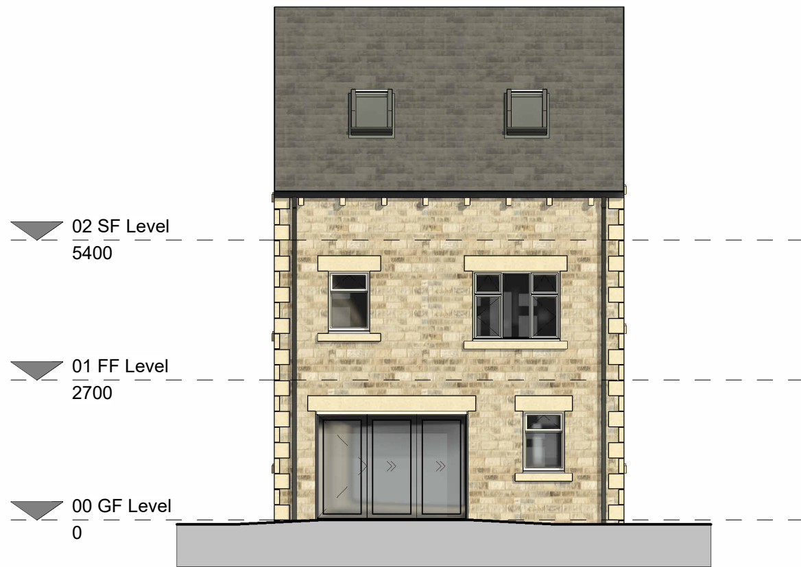
Rear 1 : 100
