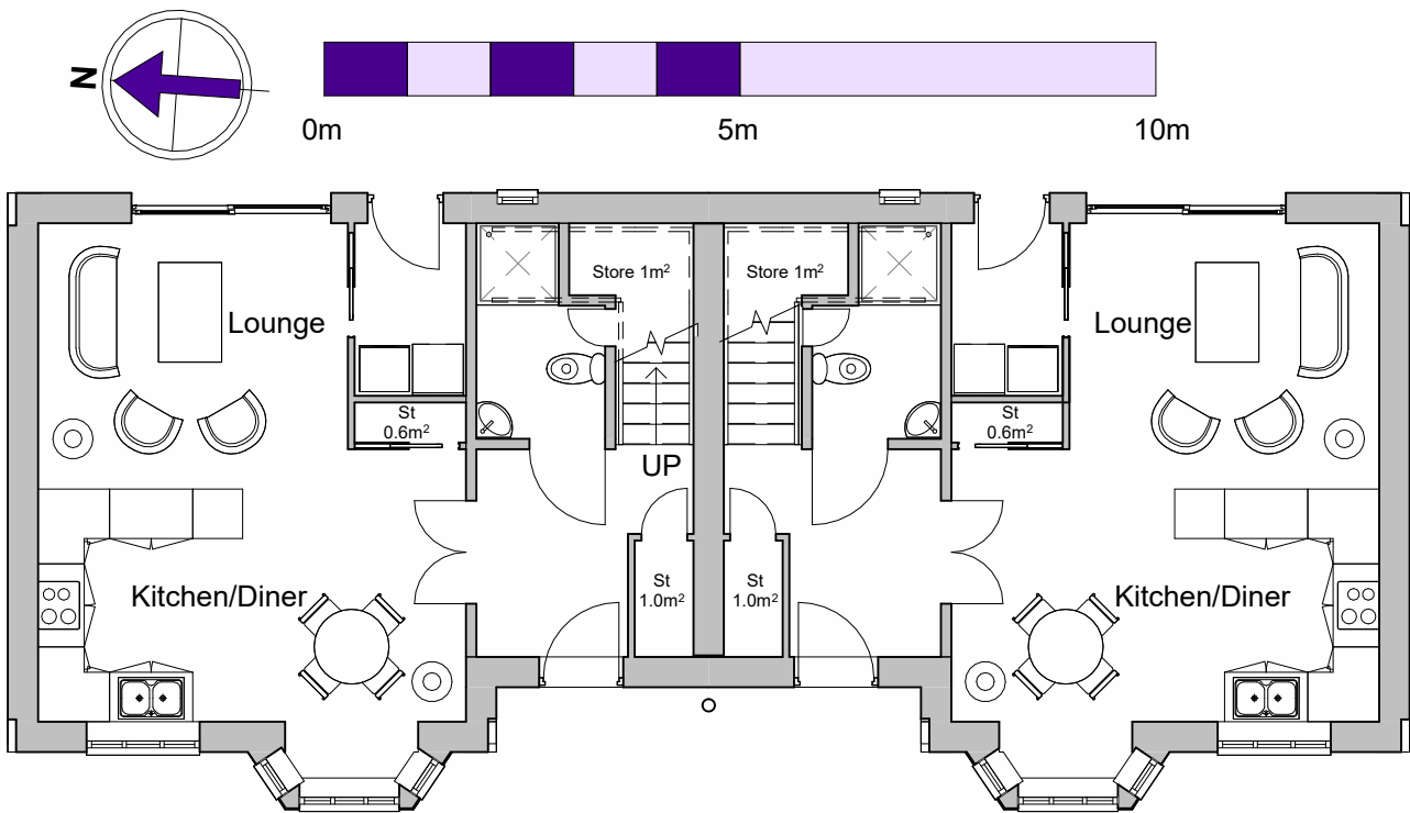
05 GFFL 1 : 100
