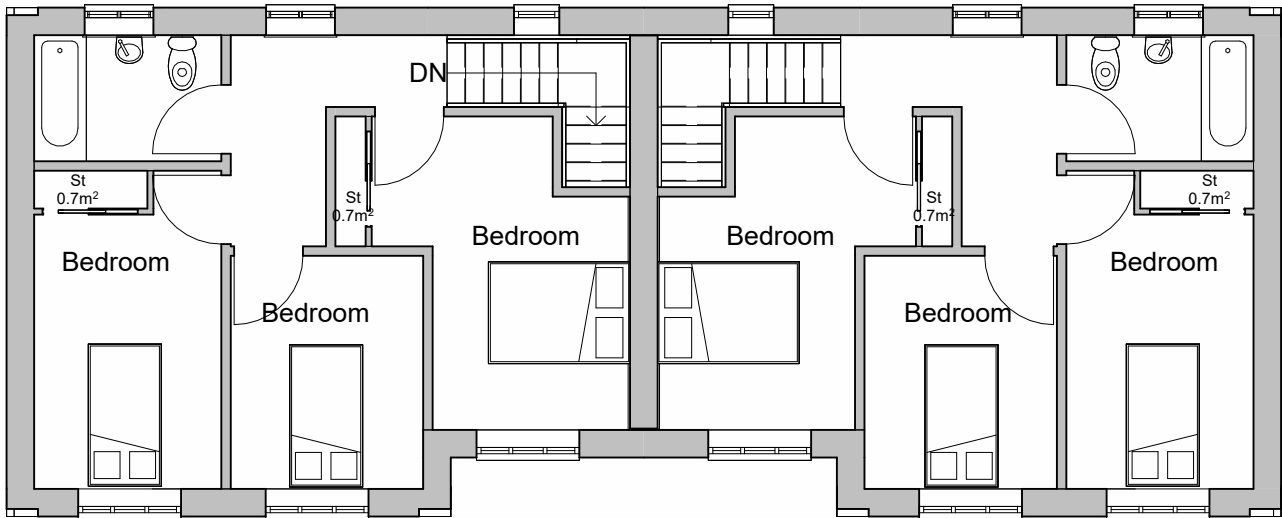
10 1FFL 1 : 100
