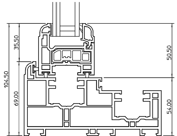
Top Jamb
