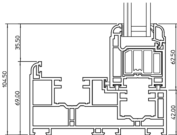
Bottom Jamb
