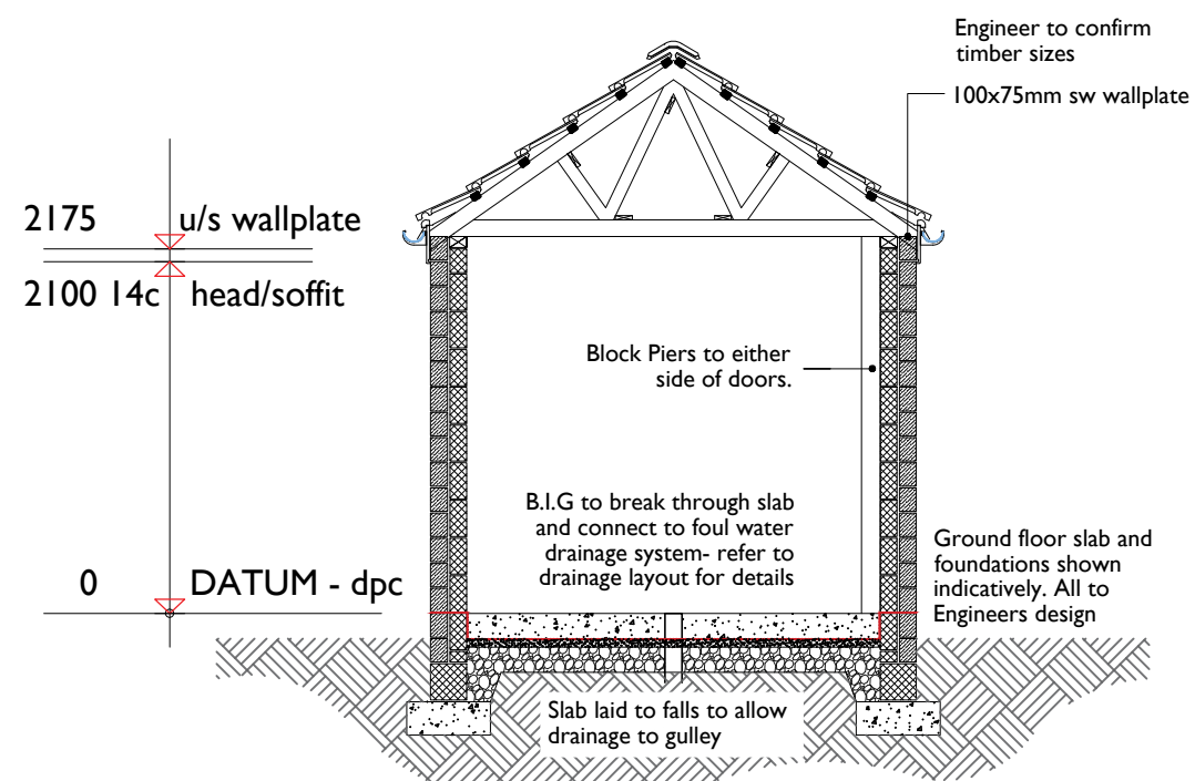
Section A-A 1:50
