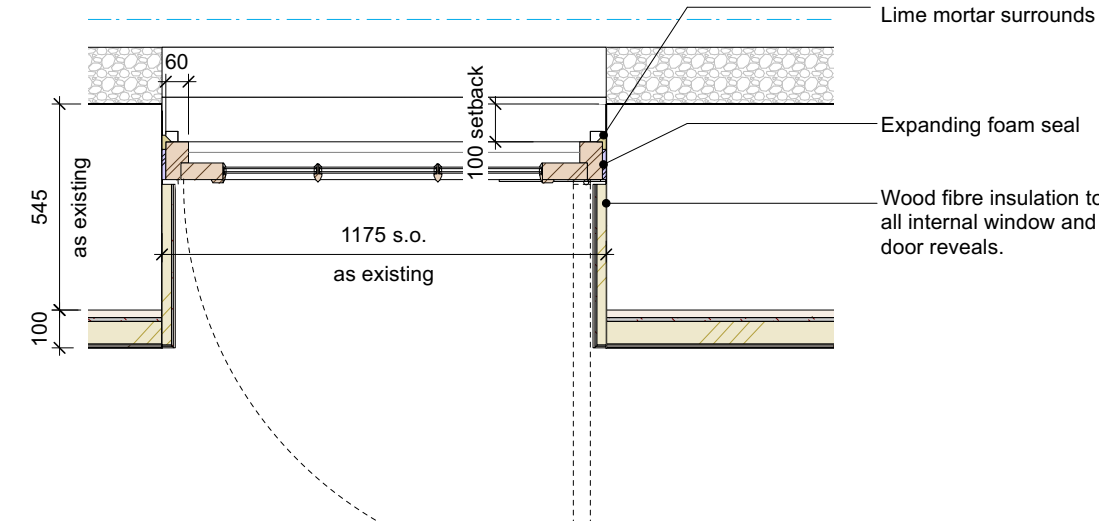
Jamb Detail Scale - 1:20
