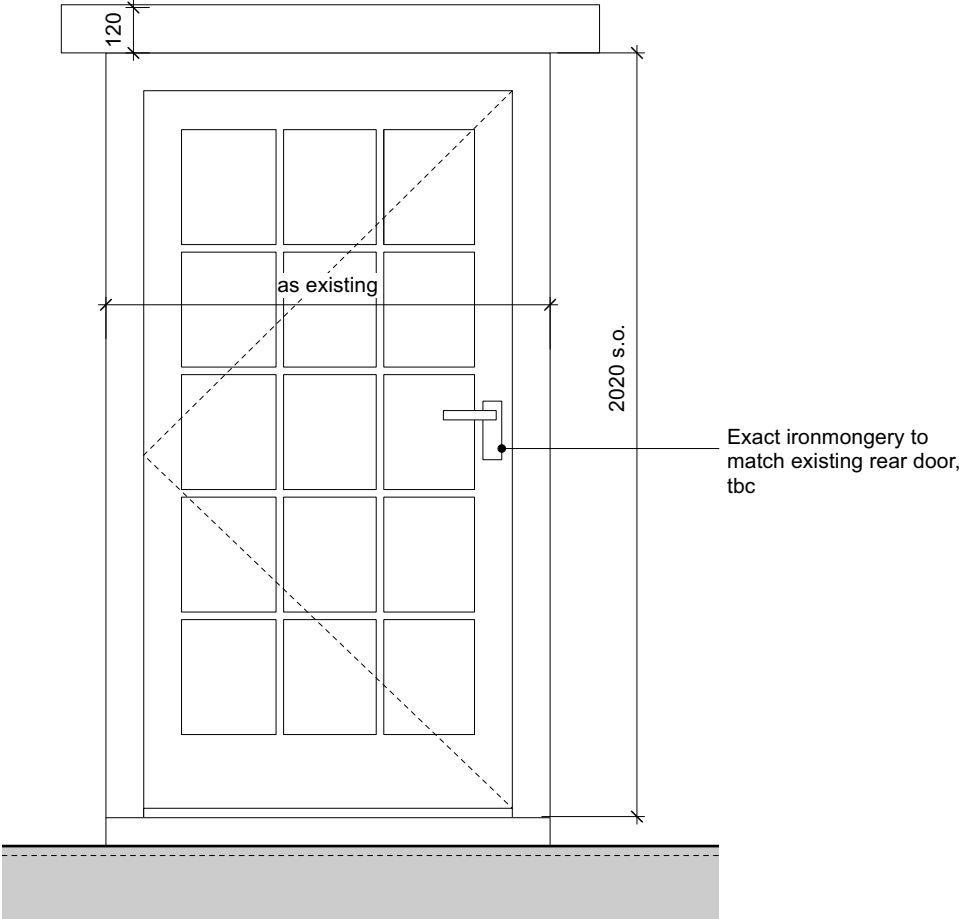
Door Elevation Scale - 1:20
