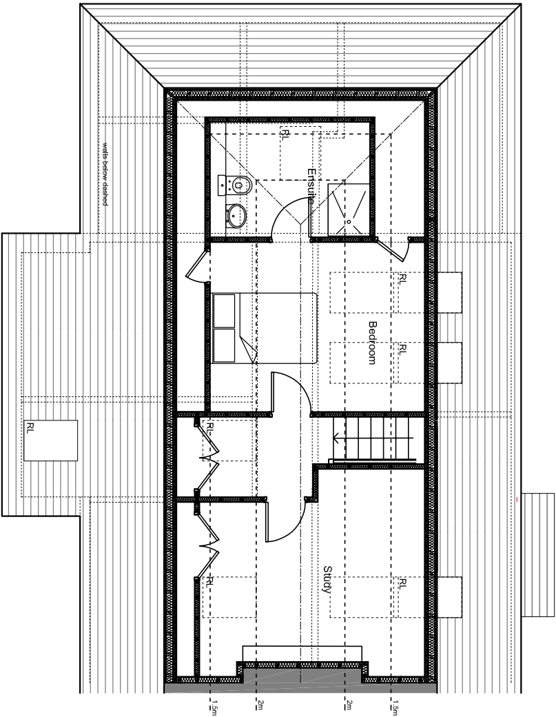
Loft
