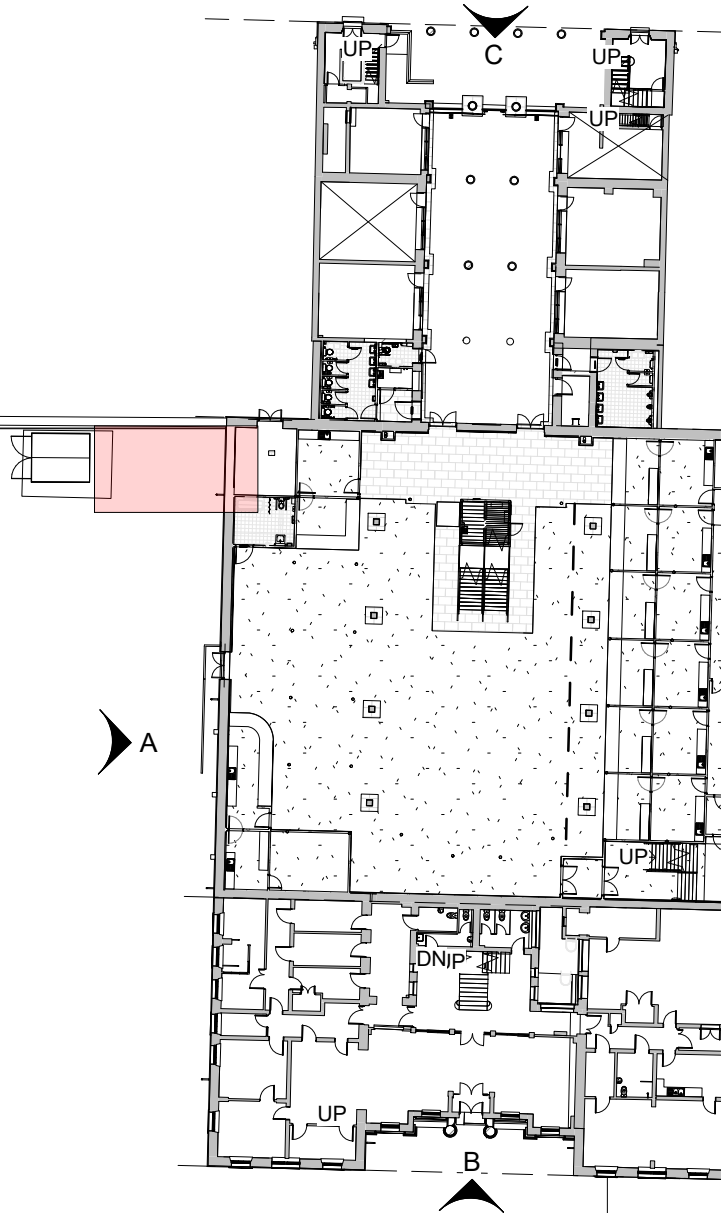
Key Plan 1 : 500
