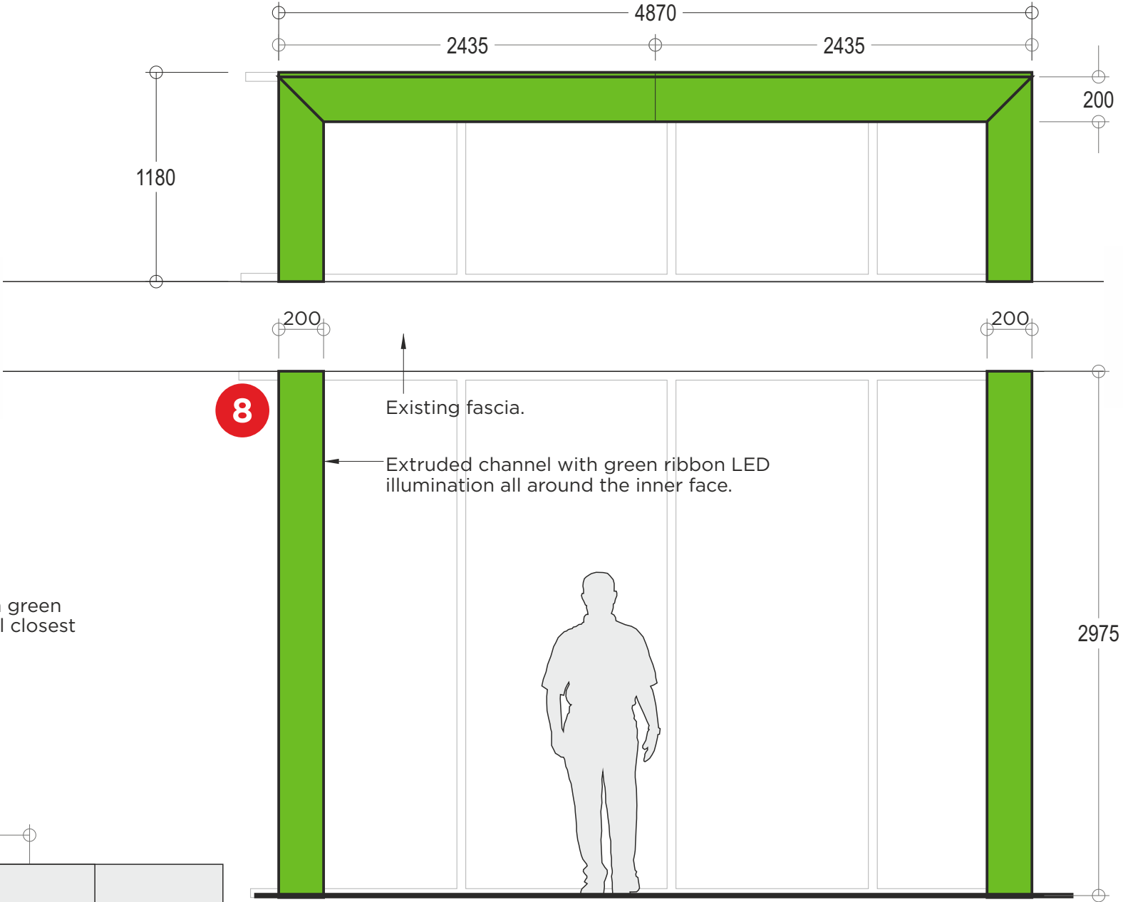
Face 1:30
