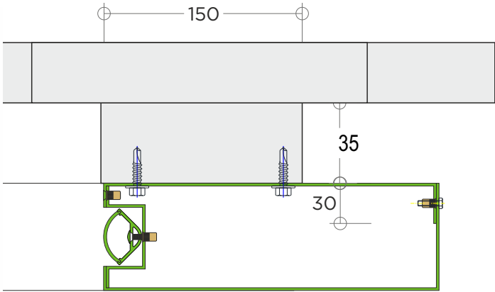
Right Section 1:4
