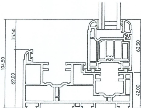
Side Jamb
