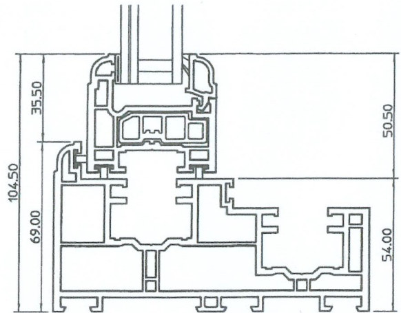
Top Jamb
