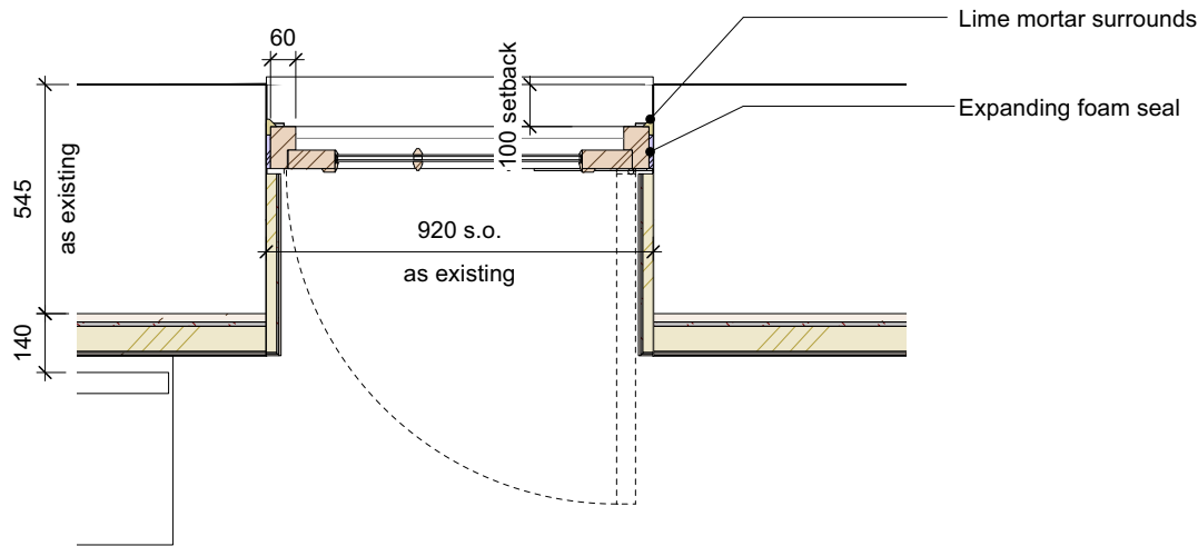
Jamb Detail Scale - 1:20
