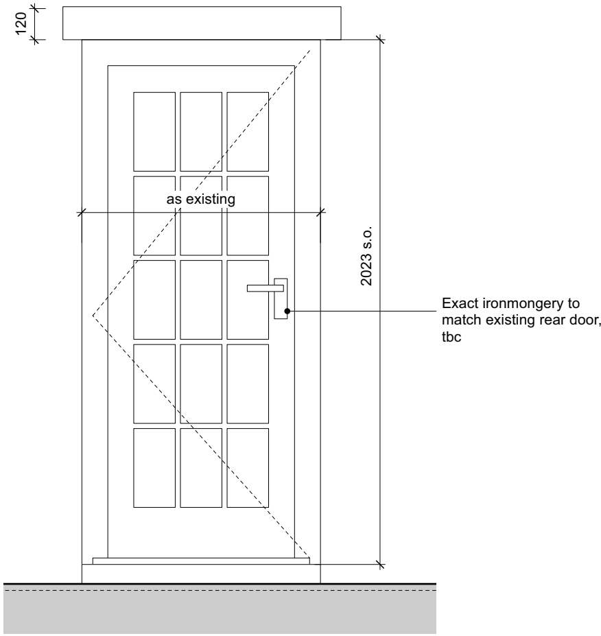
Door Elevation Scale - 1:20
