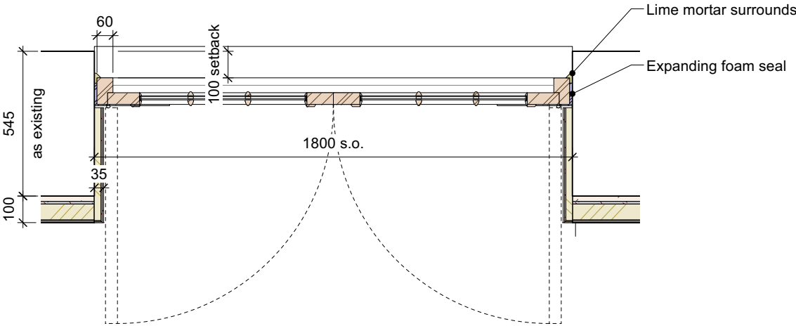
Jamb Detail Scale - 1:20
