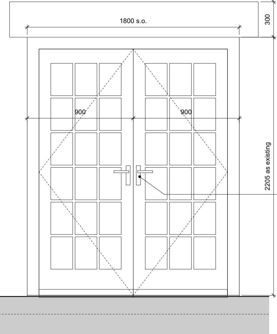
Door Elevation Scale - 1:20
