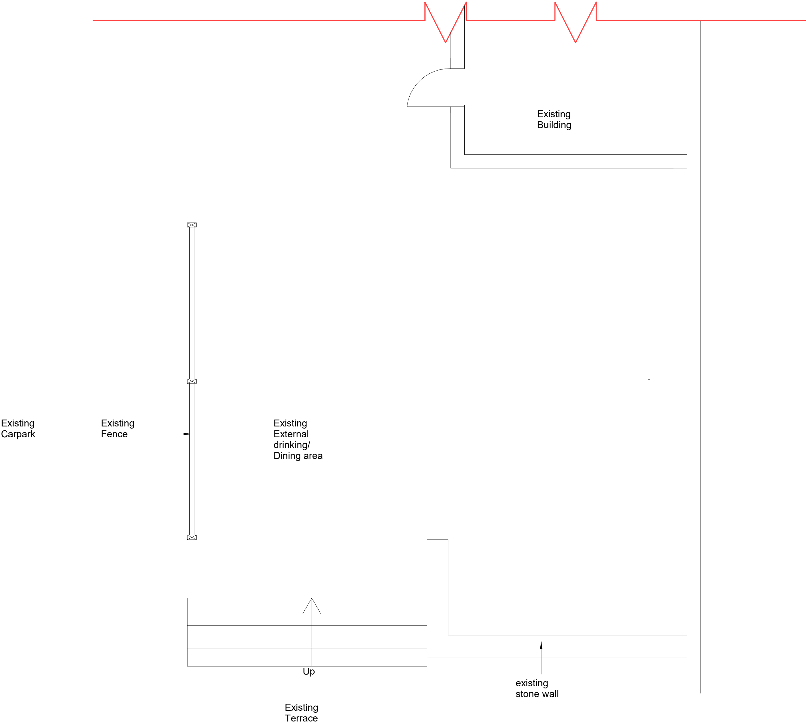
Existing Plan 1 : 50
