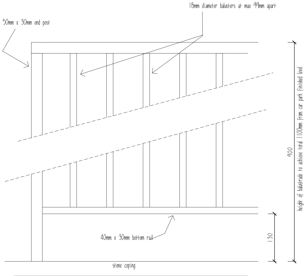
Elevation
