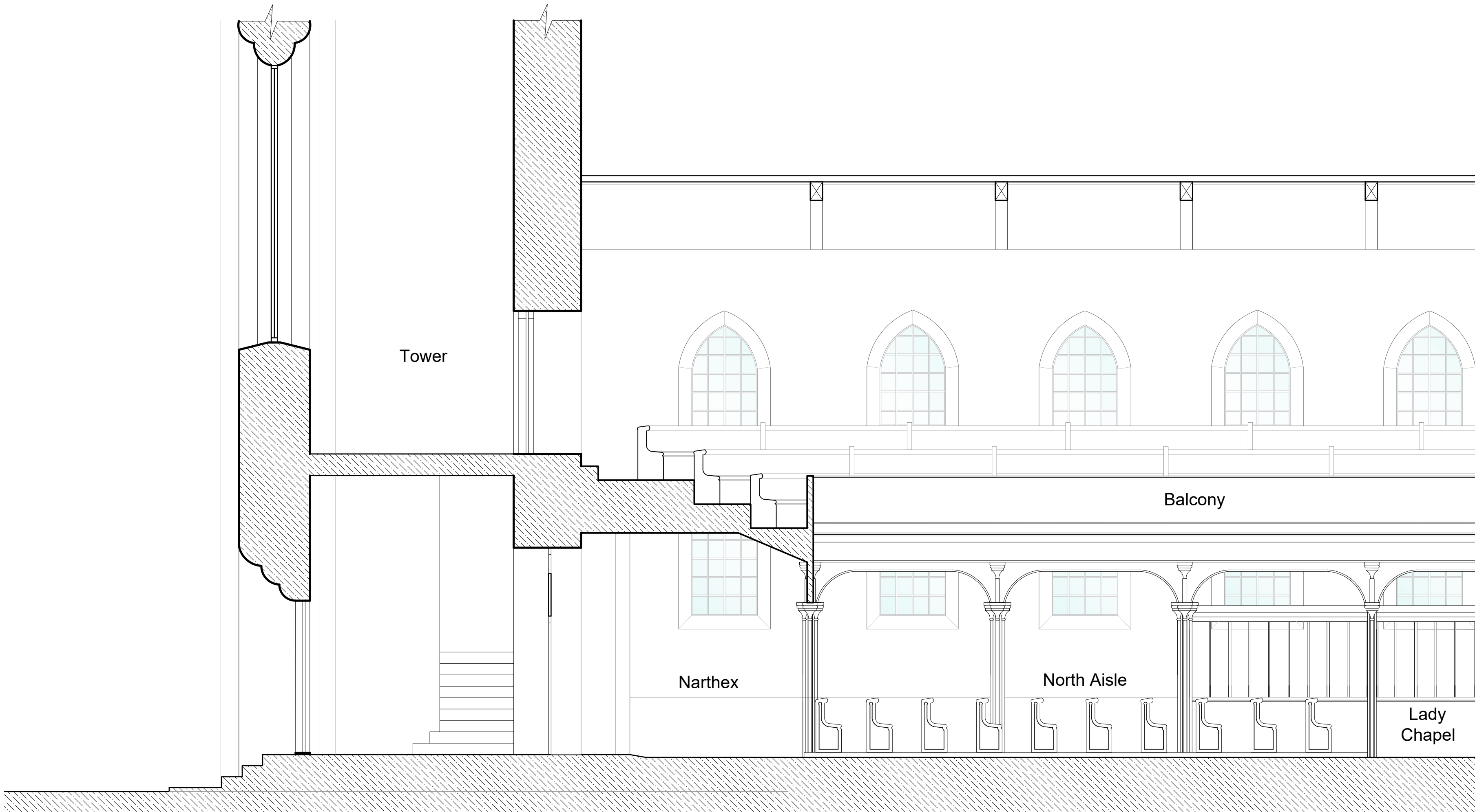
Section A-A (Scale 1:50)
