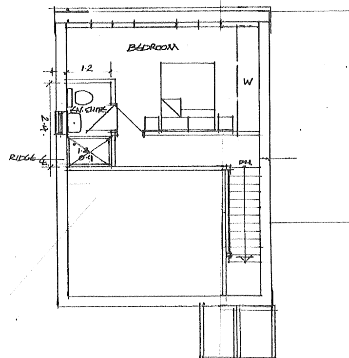
LOFT PLAN.
